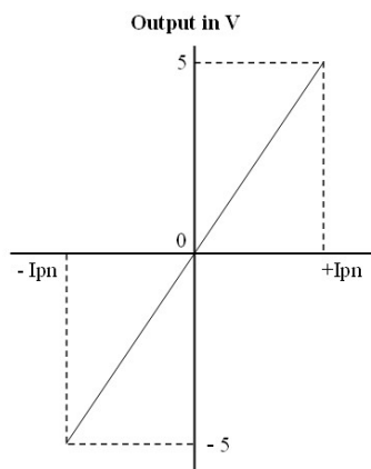
(图 2: 0±5V 输出)
