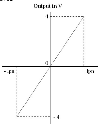
(图 1: 0±4V 输出)
